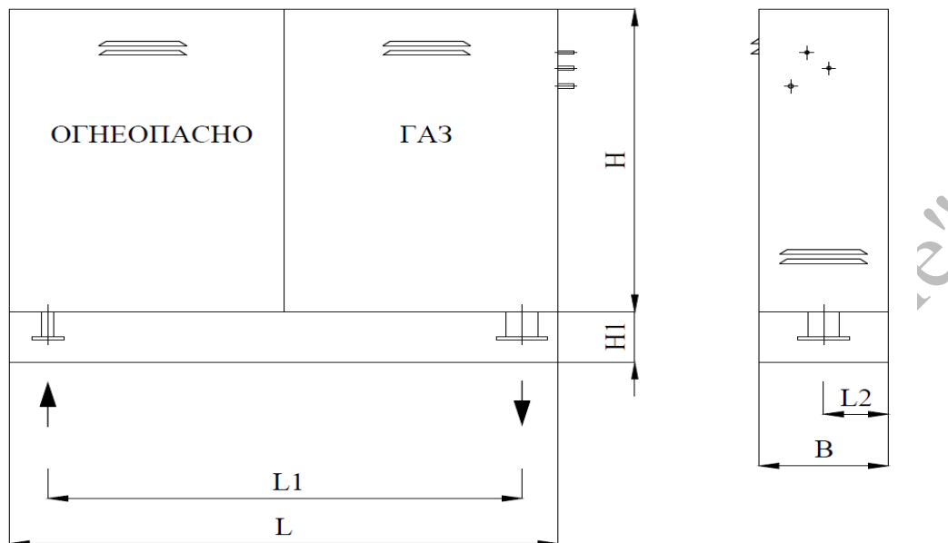
Рисунок В.2.1 – Габаритный чертеж ГРПШ. Исполнение 1
